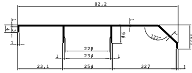
ALÜMİNYUM SÜPÜRGELİK PROFİLİ Aluminum Skirting Profile
