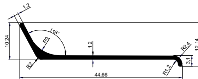
ALÜMİNYUM SÜPÜRGELİK PROFİLİ Aluminum Skirting Profile
