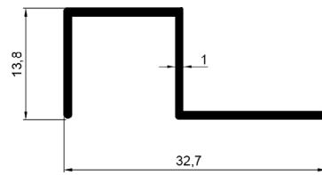
ALÜMİNYUM KARE KÖŞE FAYANS PROFİLİ Aluminum Square Corner Tile Profile
