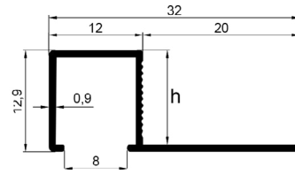
ALÜMİNYUM KARE KÖŞE FAYANS PROFİLİ Aluminum Square Corner Tile Profile
