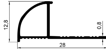
ALÜMİNYUM FEDERLİ ALT VE ÜST TIRNAKLI DIŞ KÖŞE FAYANS PROFİLİ With Aluminum Federated Top And Bottom Tabs Exterior Corner Tile Profile
