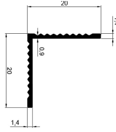
ALÜMİNYUM L MERDİVEN ÇİZGİLİ BASAMAK PROFİLİ Aluminum L Ladder Stripes Step Profile
