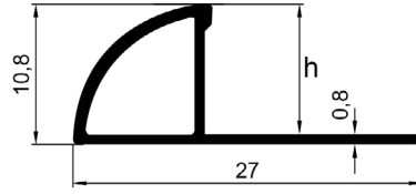
ALÜMİNYUM FEDERLİ DIŞ KÖŞE FAYANS PROFİLİ Aluminum Federated Exterior Corner Tile Profile
