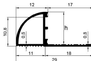
ALÜMYUM LÜKS FEDERLİ DIŞ KÖŞE FAYANS PROFİLİ Aluminum Luxury Federated Exterior Corner Tile Profile
