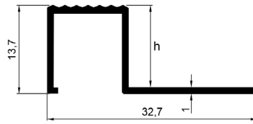
ALÜMİNYUM KARE KÖŞE FAYANS PROFİLİ Aluminum Square Corner Tile Profile
