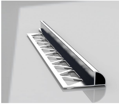
ALÜMİNYUM FEDERLİ ALT VE ÜST TIRNAKLI DIŞ KÖŞE FAYANS PROFİLİ With Aluminum Federated Top And Bottom Tabs Exterior Corner Tile Profile
