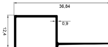
ALÜMİNYUM KARE KÖŞE FAYANS PROFİLİ Aluminum Square Corner Tile Profile
