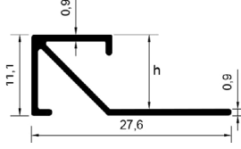
ALÜMİNYUM KARE ÇİFT TARAFLI DIŞ KÖŞE FAYANS PROFİLİ Aluminum Square Double-Sided Outer Corner Tile Profile
