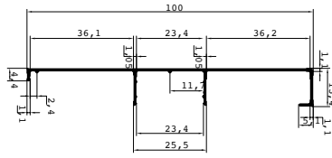
ALÜMİNYUM SÜPÜRGELİK PROFİLİ Aluminum Skirting Profile
