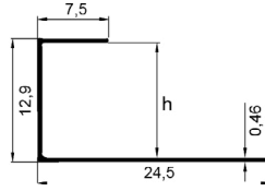
ALÜMİNYUM KARE DIŞ KÖŞE FAYANS PROFİLİ Aluminum Square Exterior Corner Tile Profile
