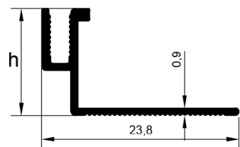
ALÜMİNYUM FAYANS GENLEŞME PROFİLİ Aluminum Tile Expansion Profile
