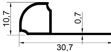
ALÜMYUM FEDERLİ DIŞ KÖŞE FAYANS PROFİLİ Aluminum Federated Exterior Corner Tile Profile
