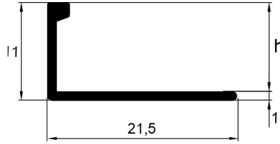
ALÜMİNYUM ÜST TIRNAKLI LÜKS FAYANS BİTİM PROFİLİ Luxury With Aluminum Top Tabs Tile Finishing Profile
